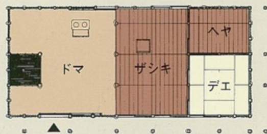
復元平面図
